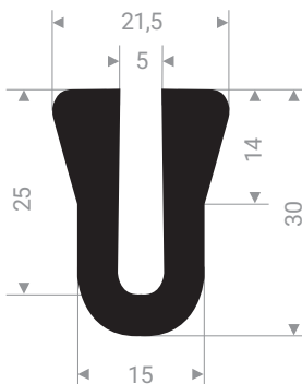
21100570 EPDM 70 Shore A noir
