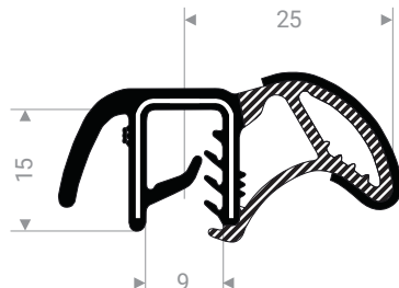
24500121 PVC + caoutchouc mousse noir plage de serrage 9 mm
