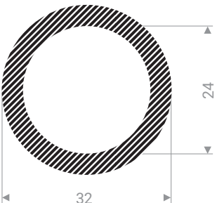
22202432 EPDM 15 Shore A noir
