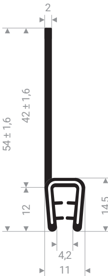
24500888 PVC + caoutchouc plein noir plage de serrage 4 - 5 mm
