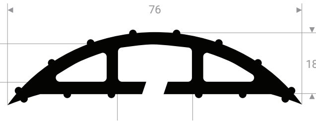
21500471 PVC 70 Shore A noir
