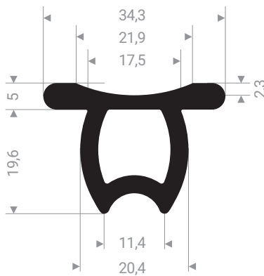
21605680 EPDM 70 Shore A noir
