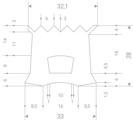
21501395W EPDM 65 Shore A blanc
