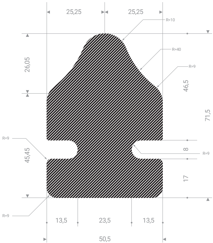
22505070 EPDM 25 Shore A noir
