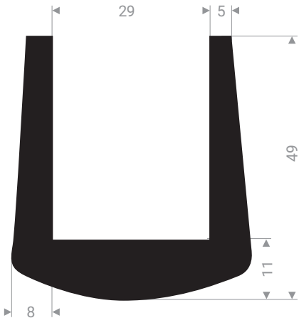
21105511 EPDM 70 Shore A noir
