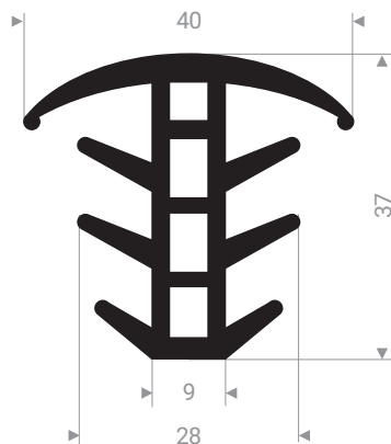
21605705 EPDM 70 Shore A noir
