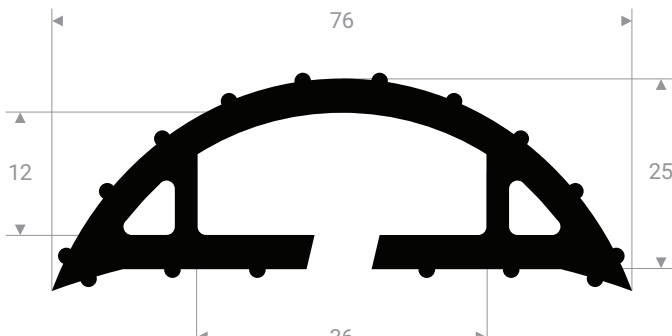
21500472 PVC 70 Shore A noir
