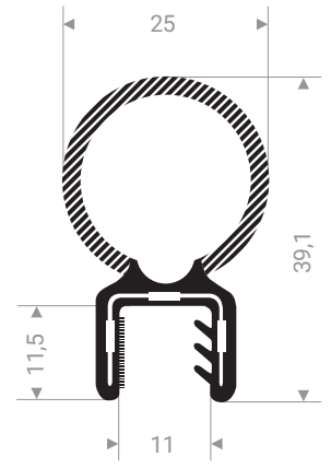
24500812 PVC + caoutchouc mousse noir plage de serrage 9 - 10,5 mm
