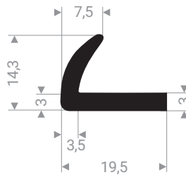
21651914 EPDM 70 Shore A noir
