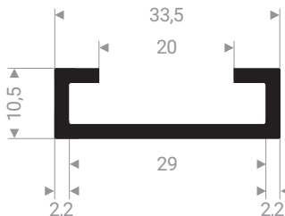
21604111 EPDM 70 Shore A noir
