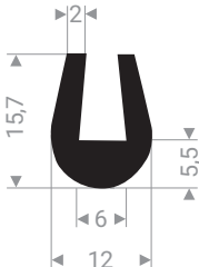
21104520 EPDM 70 Shore A noir
