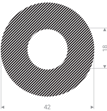
22201842 EPDM 15 Shore A noir
