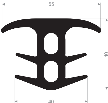
21605800 EPDM 70 Shore A noir
