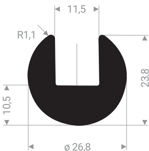
21104385 EPDM 70 Shore A noir
