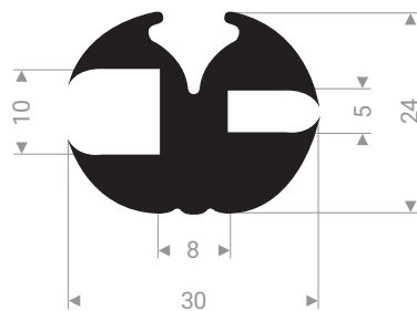
21300327 EPDM 70 Shore A noir
