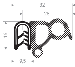
24500176 PVC + caoutchouc mousse noir plage de serrage 1 - 2 mm
