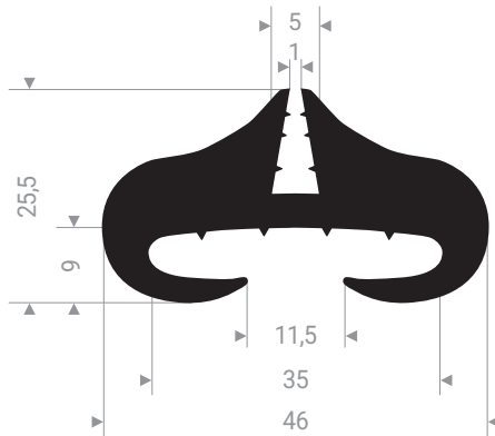
21300859 EPDM 70 Shore A noir
