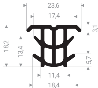
21605010 EPDM 70 Shore A noir
