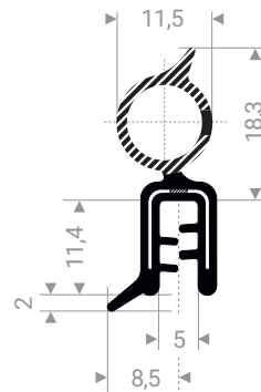
24500825 PVC + caoutchouc mousse noir plage de serrage 1,5 - 3,5 mm
