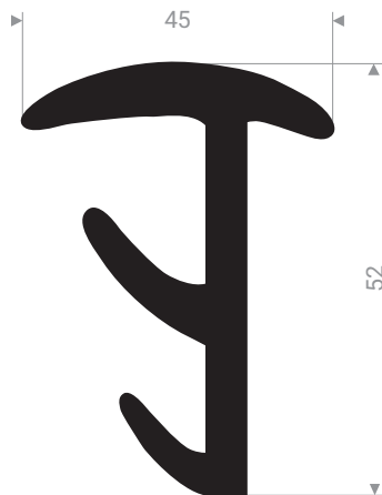
21605760 EPDM 70 Shore A noir
