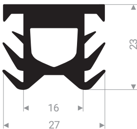
21605277 EPDM 70 Shore A noir
