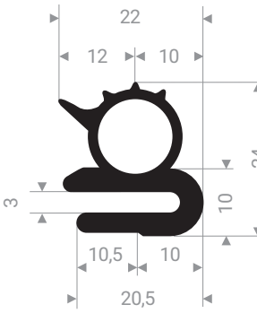
21109118 NBR 65 Shore A noir
