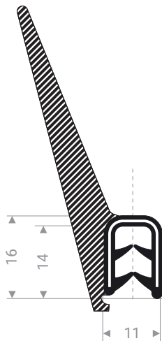
24500902 PVC + caoutchouc mousse noir plage de serrage 3 - 5 mm
