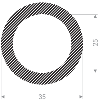
22202535 EPDM 15 Shore A noir
