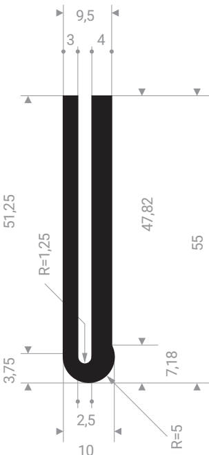
21604111 EPDM 70 Shore A noir
