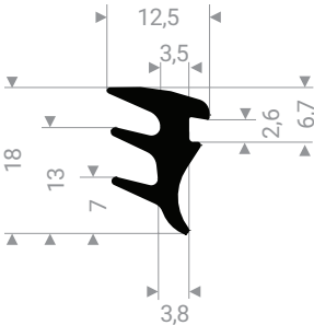
21603557 EPDM 65 Shore A noir
