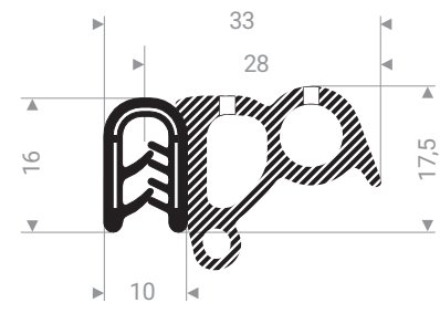
24500177 PVC + caoutchouc mousse noir plage de serrage 2,5 - 4 mm
