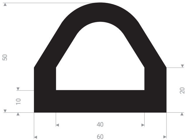
21506050 EPDM 70 Shore A noir
