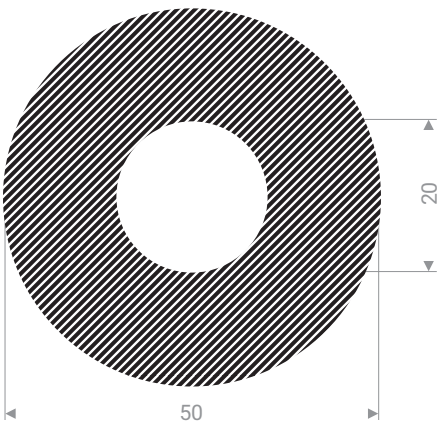
22205020 EPDM 15 Shore A noir
