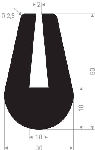
21105381 EPDM 70 Shore A noir
