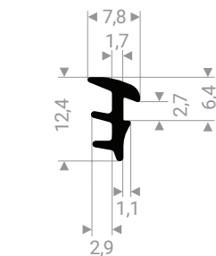
21603545 EPDM 65 Shore A noir
