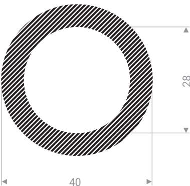
22202840 EPDM 15 Shore A noir
