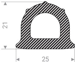
22502521 EPDM 15 Shore A noir
