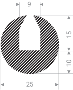
22101825 EPDM 15 Shore A noir
