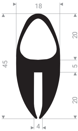
21109004 EPDM 70 Shore A noir
