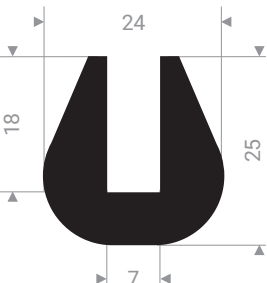
21100575 EPDM 70 Shore A noir
