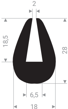
21100565 EPDM 70 Shore A noir
