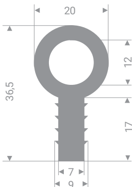
21603101GR EPDM 70 Shore A gris
