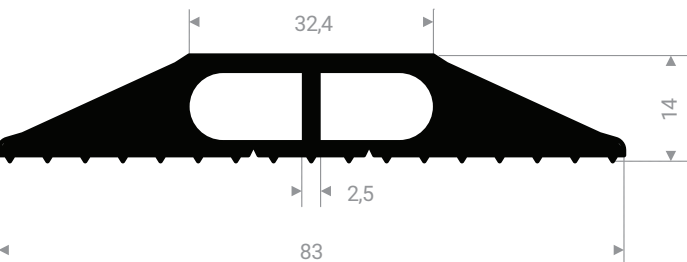
21500485 EPDM 70 Shore A noir
