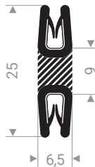
24100555 PVC + plastique noir plage de serrage 0,5 - 1,5 mm
