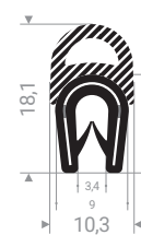
24500817 PVC + caoutchouc mousse noir plage de serrage 1,5 - 3 mm
