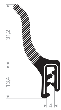
24500920 PVC + caoutchouc mousse noir plage de serrage 1,5 - 4 mm
