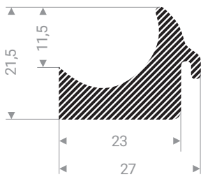
22500752 EPDM 15 Shore A noir
