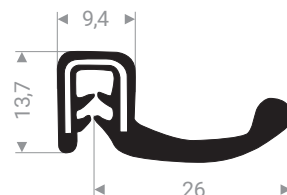
24500315 PVC + caoutchouc plein noir plage de serrage 1,5 - 4 mm
