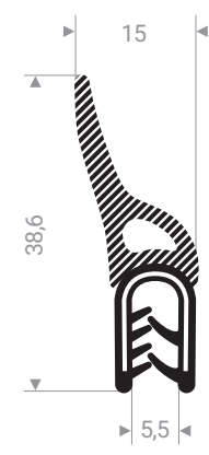
24500935 PVC + caoutchouc mousse noir plage de serrage 1,5 - 3,5 mm
