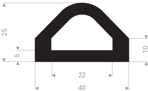
21504025 EPDM 70 Shore A noir
