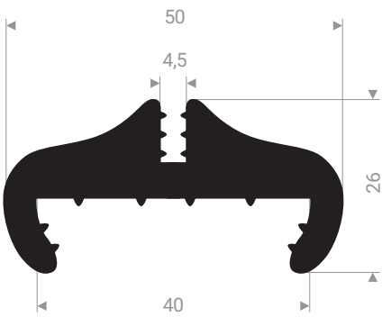
21300860 EPDM 70 Shore A noir
